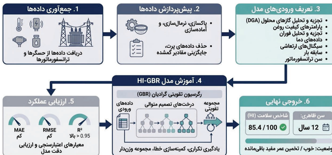
[1] شکل ۱. الگوریتم چارتهی روش پیشنهادی
