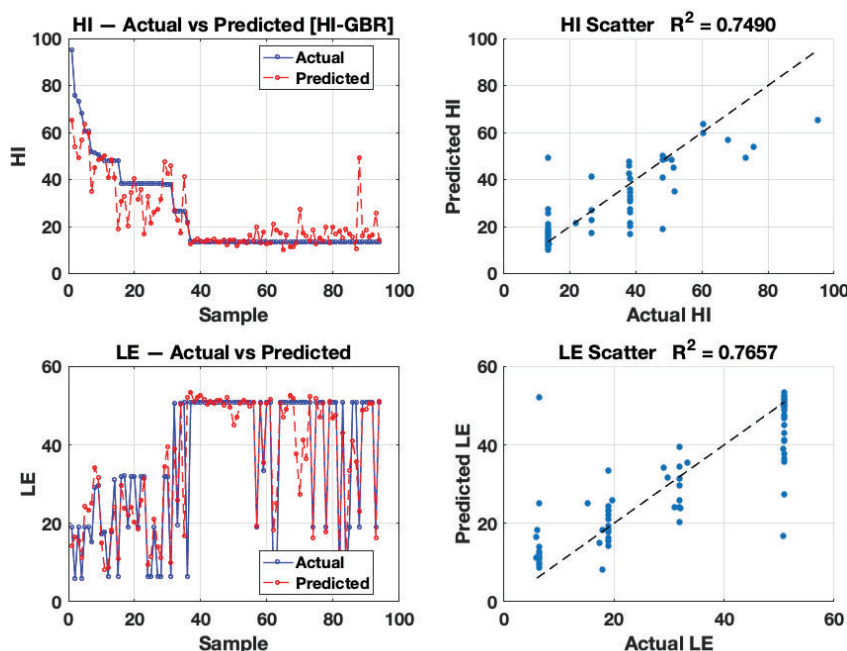
شکل ۲. نتایج حاصل از اعمال الگوریتم پیشنهادی بر روی داده های تست مجموعه اول
